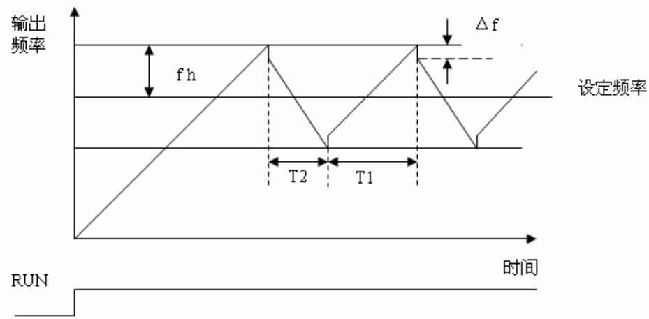
图 6.3.14 摆频运行图
