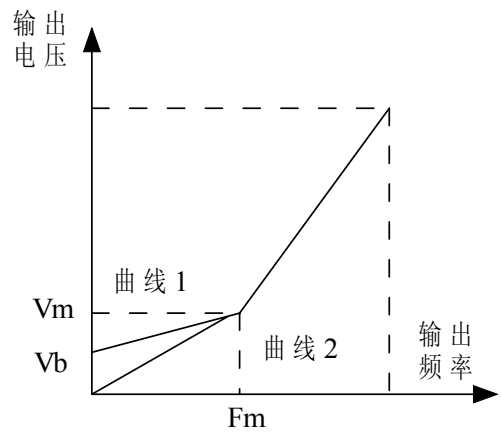
图 6.1.6 折线 V/F 曲线
