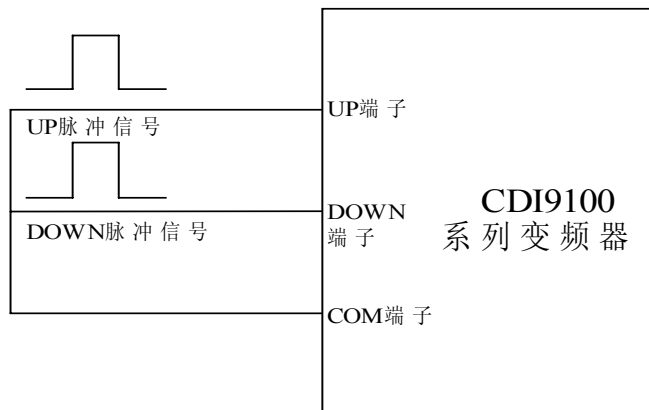
图6.1.2 频率给定8、9 方式时, 接线示意图
