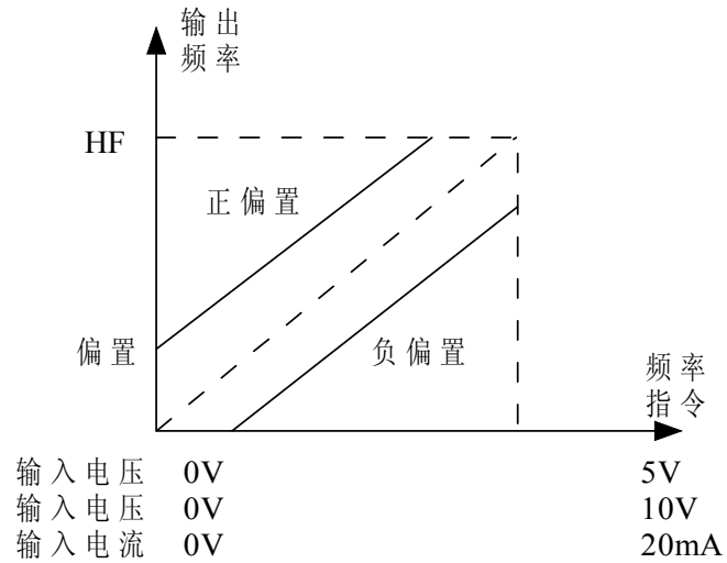
图6.2.4 偏置频率
