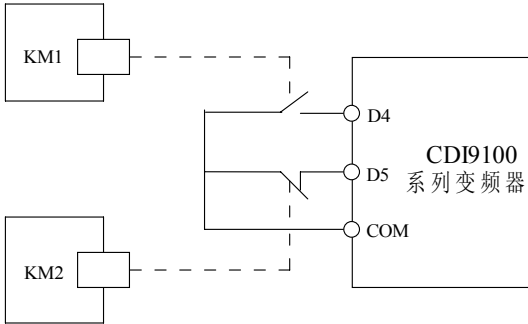
图 6.3.5 外部设备故障常开/常闭输入示意图
