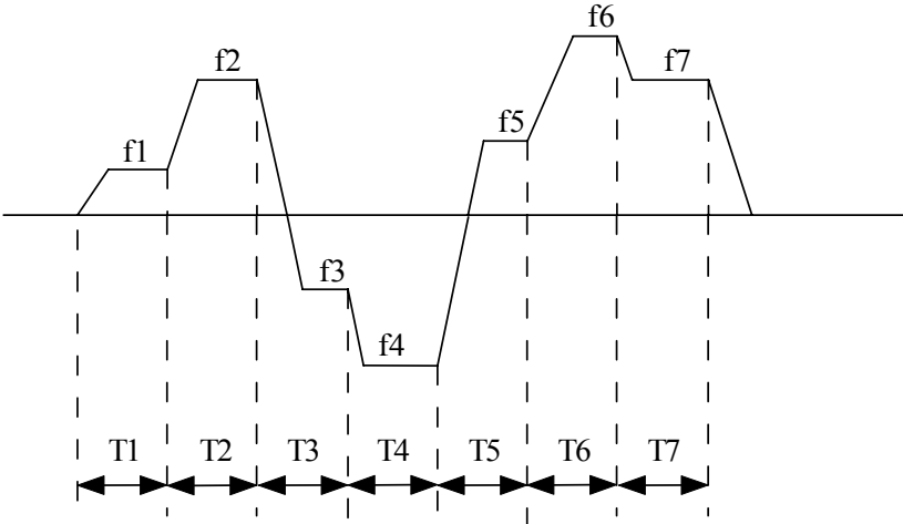
图6.3.13 可编程多段速运行示意图
