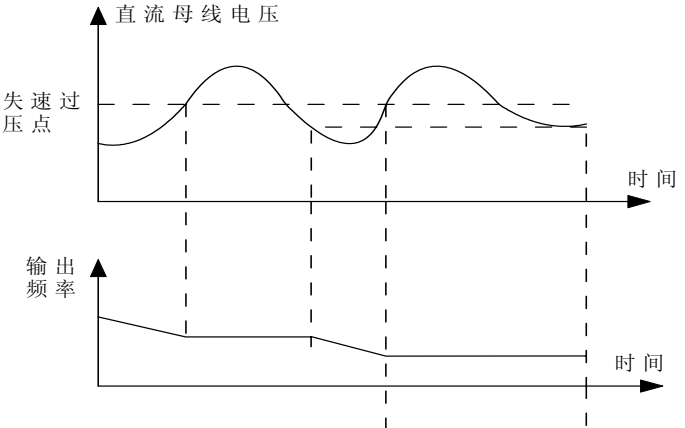
图6.4.1 过压失速功能示意图
