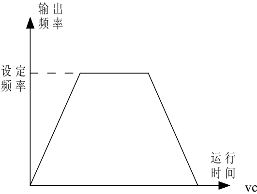
图 6.1.7 直线加减速
