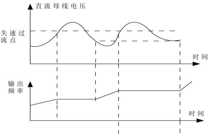
图6.4.2 失速过流保护
