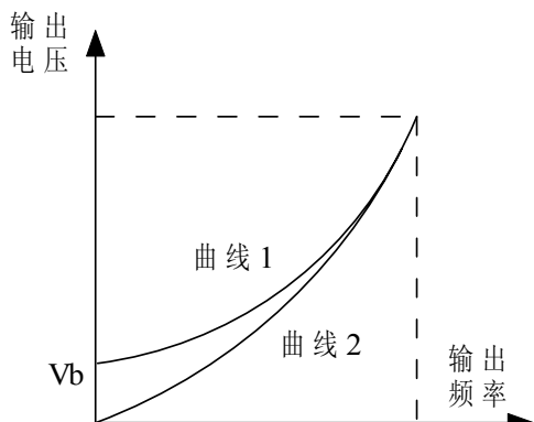
图 6.1.4 递减转矩模式 1
