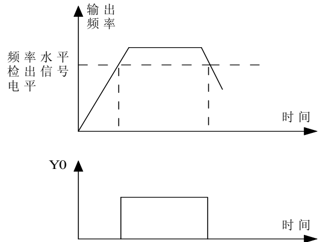
图6.3.11 频率水平检出信号示意图
