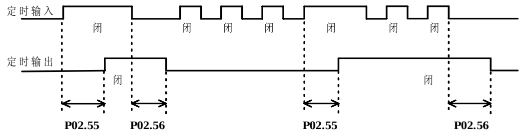
图 6.3.15 定时器功能图
