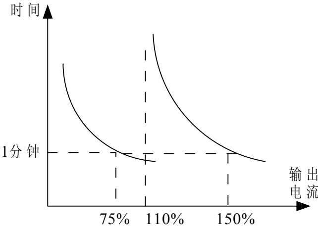
图6.1.12 过载保护反时限特性曲线
