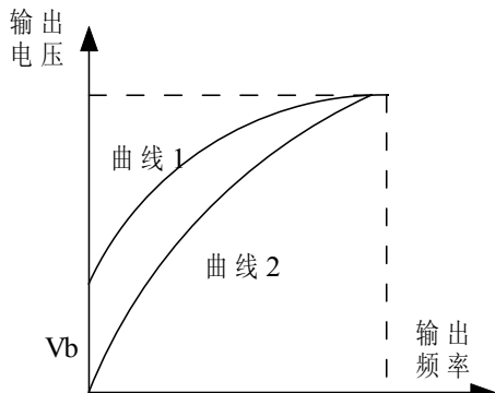
图 6.1.5 递减转矩模式 2
