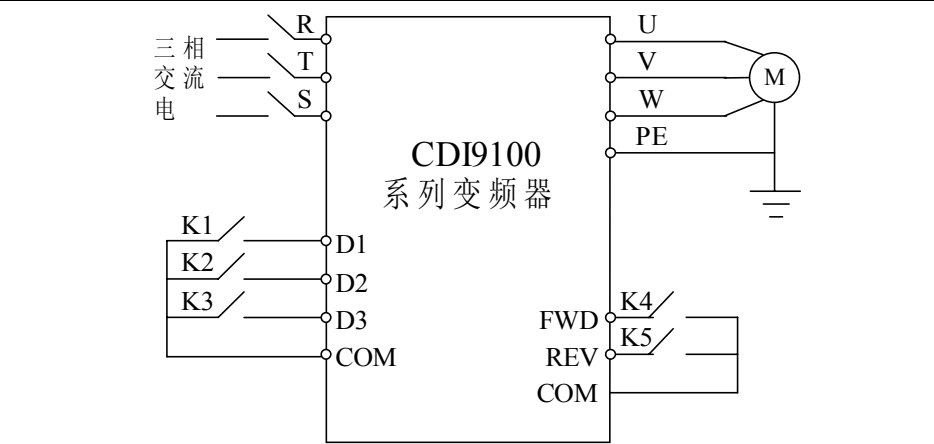
图6.3.2 多段速度运行接线图
